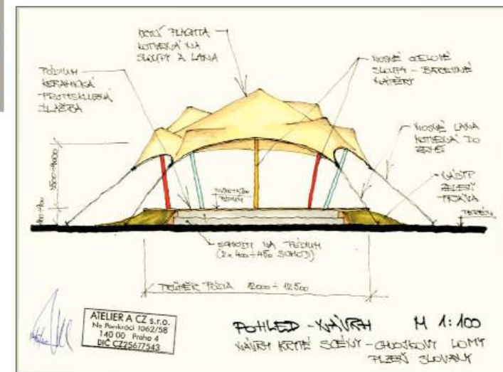
NÁVRH ZASTŘEŠENÍ - POHLED JIŽNÍ
